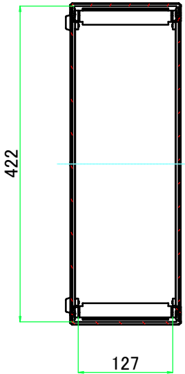
A-A ( 1 : 7 )
